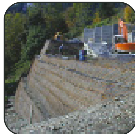
Verbier, Schweiz: Rückverhängte Gabionenwand mit Enkagrid PRO 40
